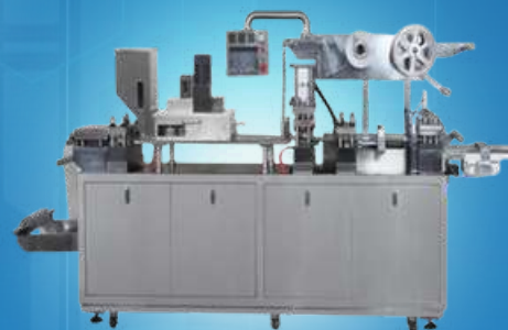
เครื่องบรรจุแผงบลิสเตอร์
